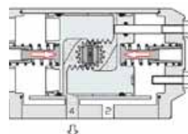
4: outlet air
